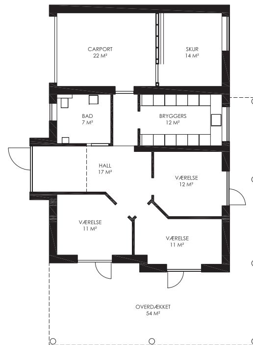
PRIMA GRUNDPLAN - 92 M 2 GARAGE 42 M 2
