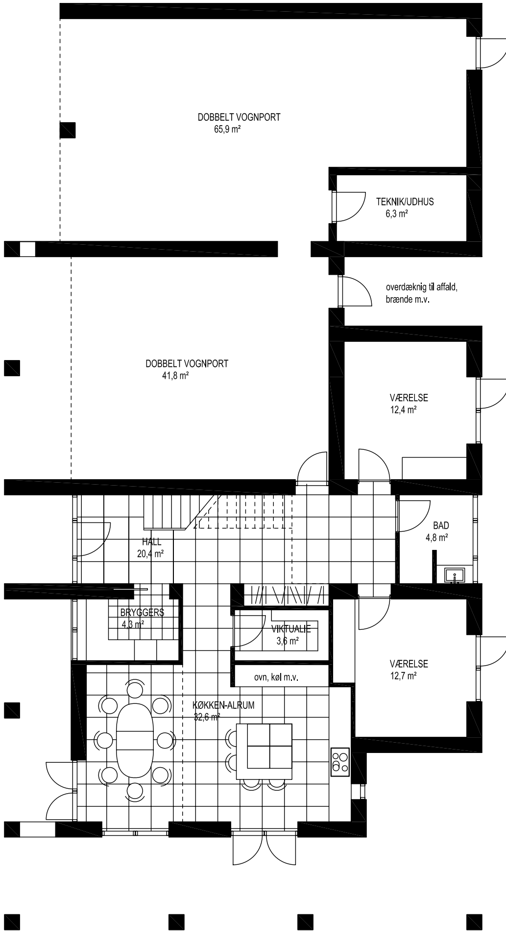
STUEPLAN BRUTTOETAGEAREAL 114 m 2
